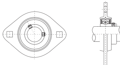
Supporto in lamiera stampata BPP
