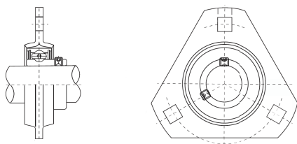
Supporto in lamiera stampata BPFL
