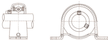
Supporto in lamiera stampata BPFL
